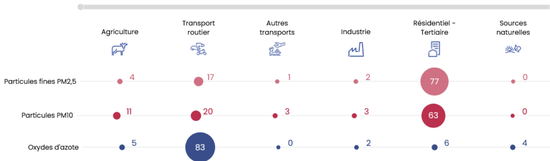
Contribution des activités humaines et naturelles aux émissions de polluants atmosphériques (%) pour l'année 2022
