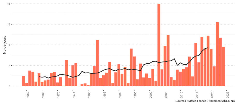
Nouvelle-Aquitaine - Nb nuits tropicales (t° min > 20°C) Nombre moyen de dépassements sur le territoire
