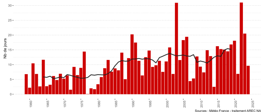
Nouvelle-Aquitaine - Nb jours avec t° max > 30°C Nombre moyen de dépassements sur le territoire
